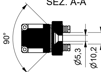
SEZ. A-A
