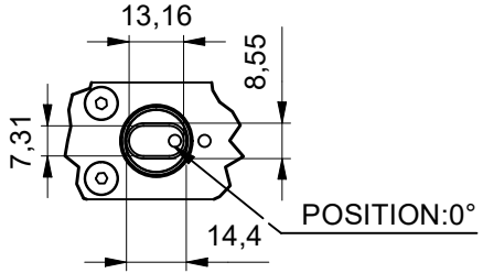
DETTAGLIO B ( 1 : 2 )
