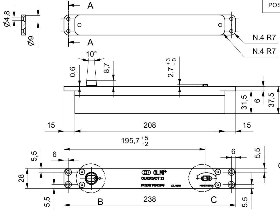
SEZ. A-A
