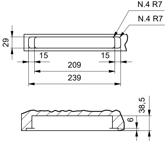
DOOR MACHINING
